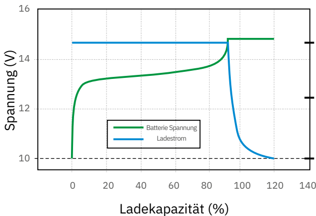
Ladeigenschaften (0,5C bei 20 °C)
